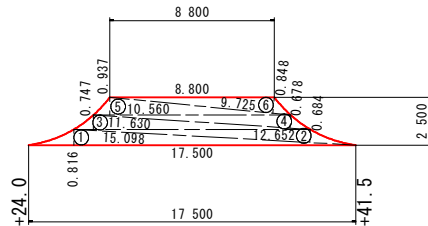
取合い1 S=1/200
