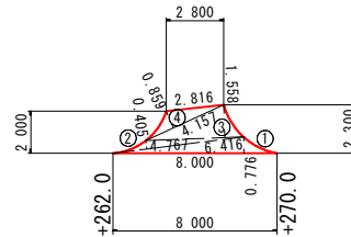
取合い3 S=1/200
